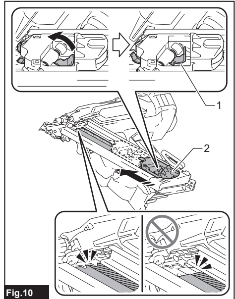
► 1. Levier-poussoir 2. Poussoir
