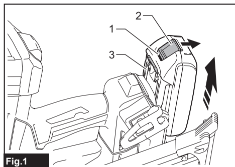
Fig.1 ▶ 1. Indicador rojo 2. Botón 3. Cartucho de batería
