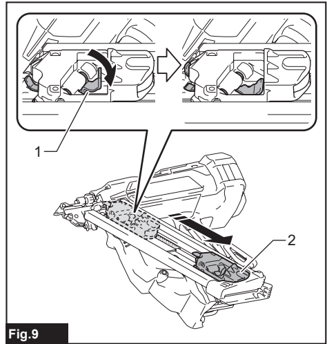
► 1. Levier-poussoir 2. Poussoir
